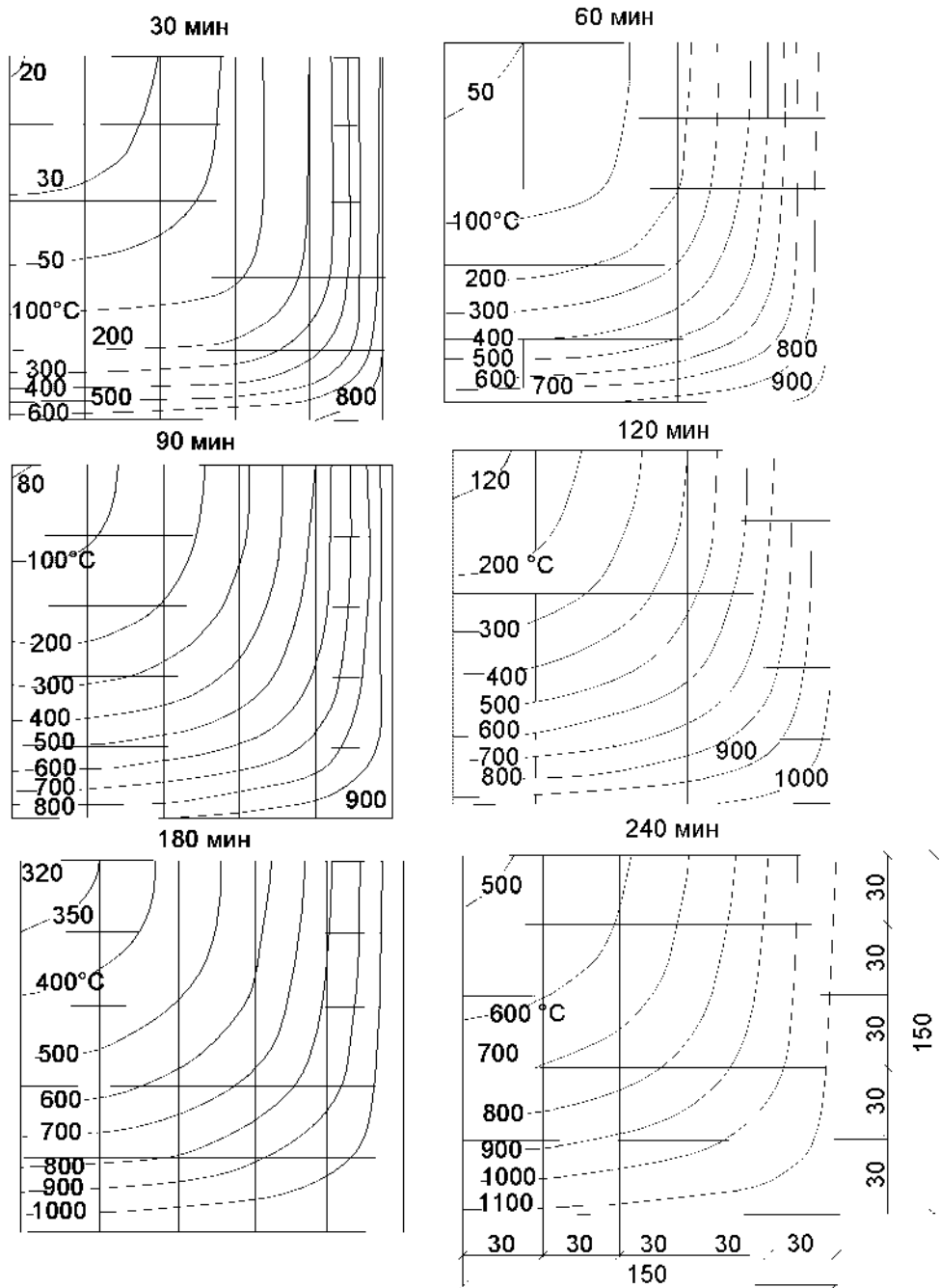
Рисунок И.1 - Колонна из тяжелого бетона сечением 300 x 300 мм при нагреве с четырех сторон
