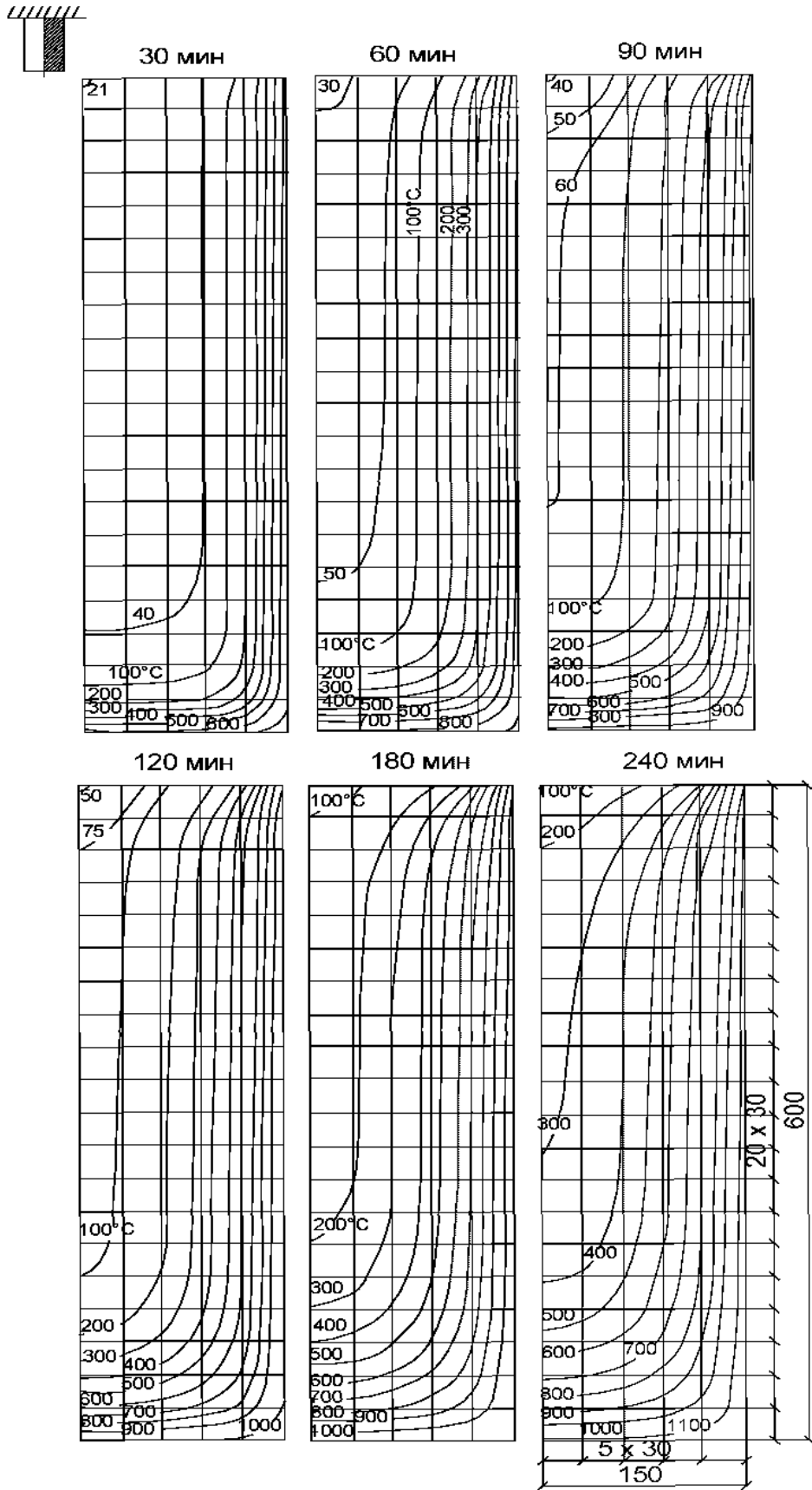
Рисунок И.7 - Балка из тяжелого бетона сечением 600 х 300 мм
