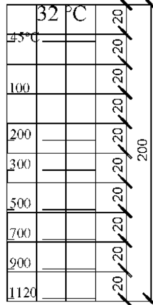
Рисунок И.15 - Плита из легкого бетона толщиной 200 мм при нагреве с одной стороны
