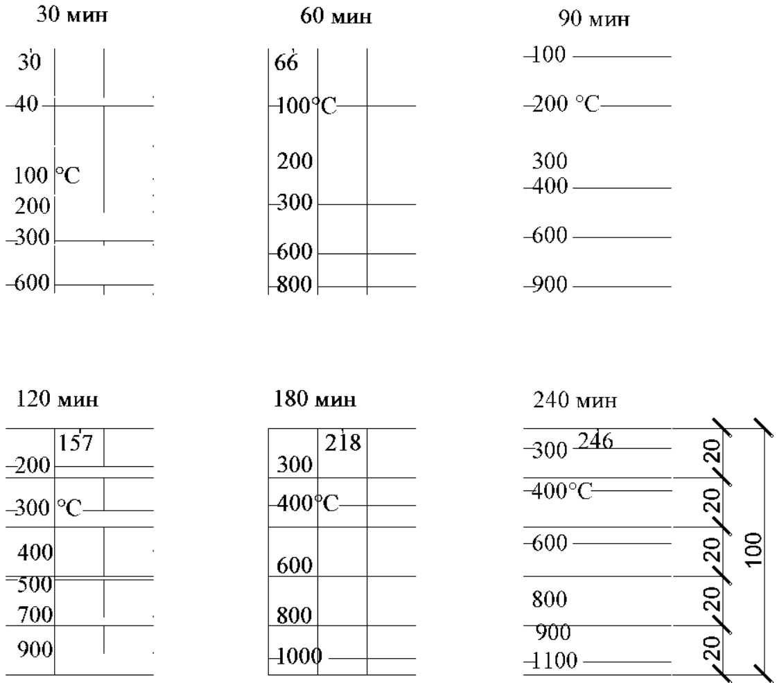
Рисунок И.11 - Плита из тяжелого бетона толщиной 100 мм при нагреве с одной стороны
