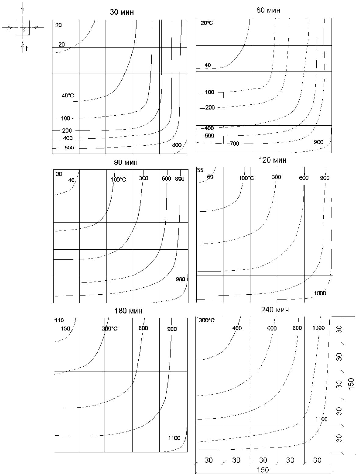
Рисунок И.3 - Колонна из легкого бетона сечением 300 x 300 мм при нагреве с четырех сторон
