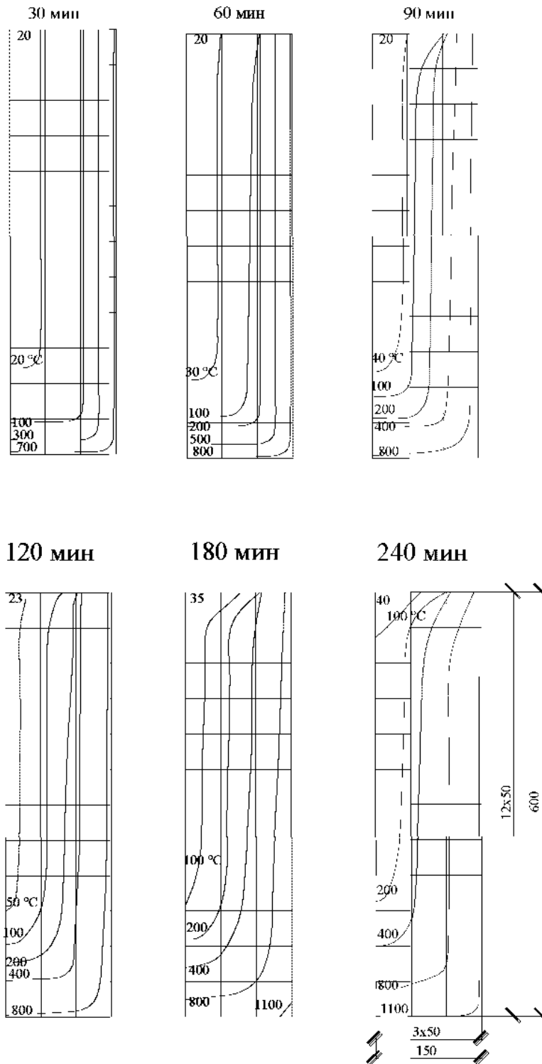
Рисунок И.10 - Балка из легкого бетона сечением 600 х 300 мм при нагреве с трех сторон
