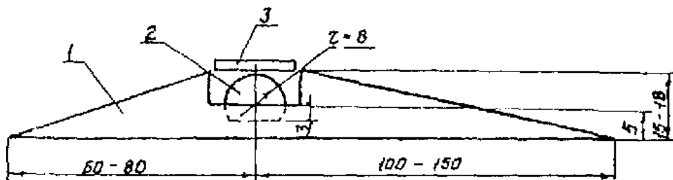
Рис. 9. Устройство для определения давления колес крана:
