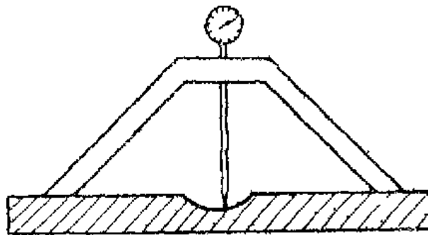
Рис. 6. Прибор Томашова
