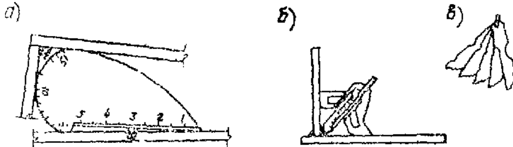
Рис. 5. Шаблоны для замера катетов швов: а - универсальный шаблон А.И. Красовского, б - универсальный шаблон В.Э. Ушера-Маршака, в - набор шаблонов
