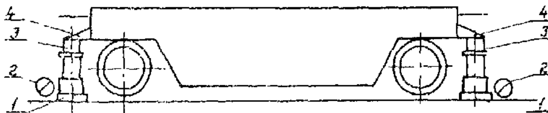
Рис. 7. Схема расположения приборов и оборудования при взвешивании крана: 1 - гидравлический домкрат, 2 - манометр, 3 - центрирующая вставка, 4 - кронштейн
