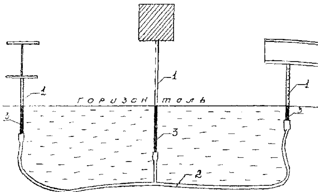
Рис. 1. Схема гидравлического нивелирования: 1 - стеклянные трубки с делениями, 2 - соединительная резиновая трубка, 3 - подкрашенная вода
