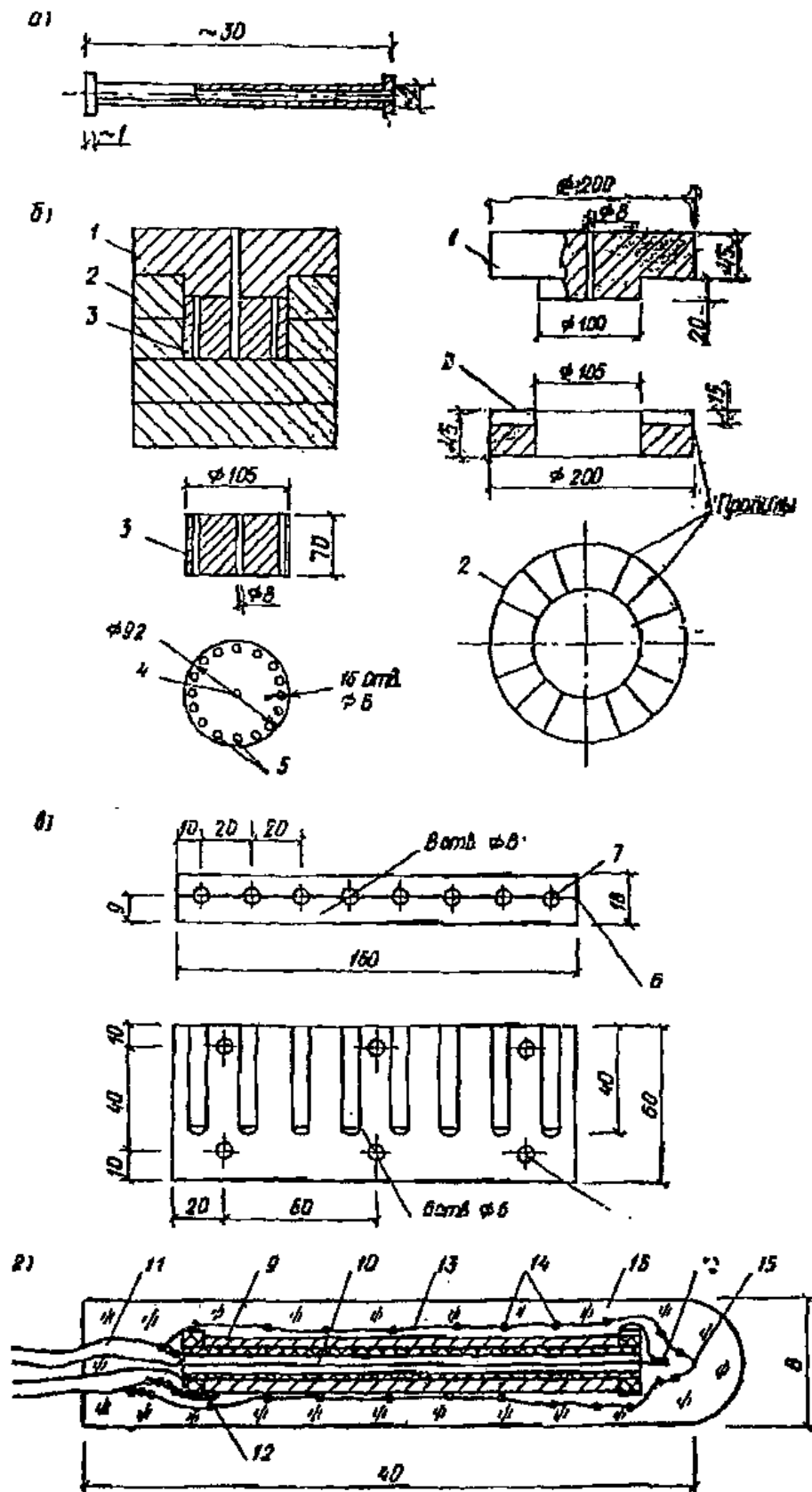
Рис. 7. Схема изготовления ЭТС а - каркас ЭТС; б - теплообменник (общий вид в разрезе и детализовка); в - форма для заливки ЭТС эпоксидной смолой (органическое стекло); г - ЭТС (показан в масштабе 3:1); 1 - крышка верхняя (пенопласт); 2 - кольцо с прорезями
