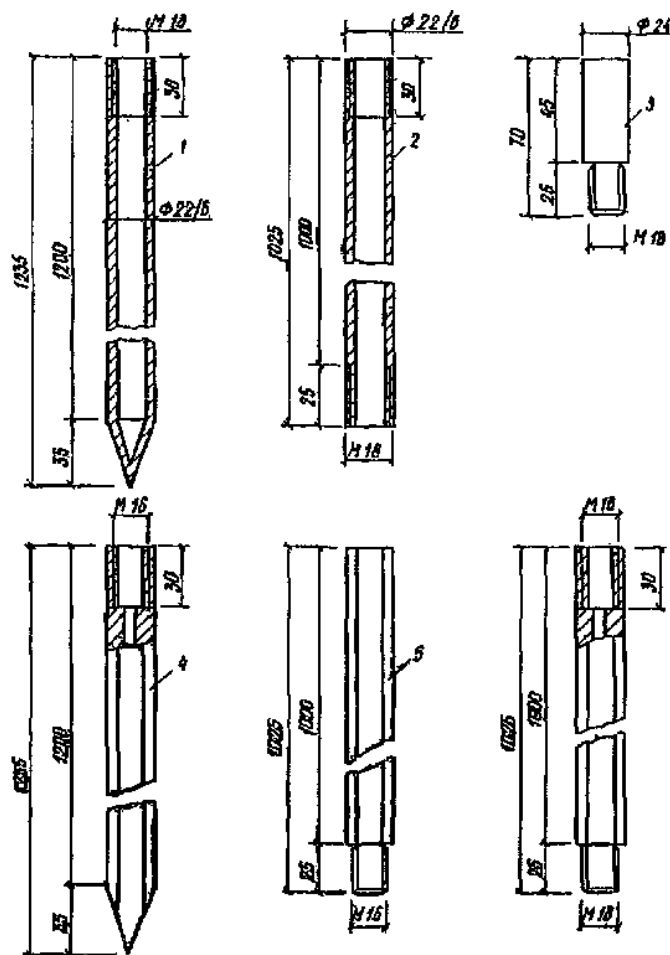
Рис. 4. Термозонд для обследований в подпольях зданий 1 - нижняя часть составной температурной трубки (труба бесшовная); 2 - верхняя часть составной температурной трубки; 3 - ударная часть, выполнена из стали марки Ст 3; 4 - нижняя часть бурового зонда (сталь буровая шестигранная 22/25); 5 - верхняя часть составного зонда
