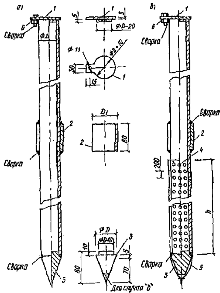
Рис. 3. Устройство контрольных температурных и гидрогеологических скважин а - обсадная труба температурной скважины; б - обсадная труба гидрогеологической скважины; 1 - защитная крышка; 2 - обойма; 3 - наконечник; 4 - отверстия по периметру трубы; 5 - латунная сетка с отверстиями \varnothing от 0,1 до 0,2 мм; 6 - приваренная к трубе гайка М 10; h - длина перфорированного участка, защищенного сеткой
