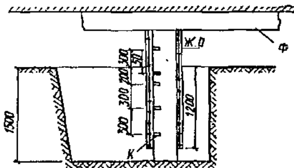
Рис. 5. Схема обследования бетона фундаментов Ф - фундаментные балки; К - место взятия керна; Ж.О - железобетонная обойма усиления фундамента
