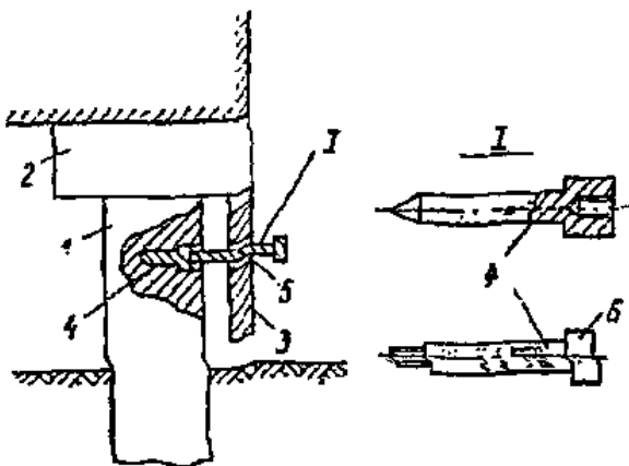
Рис. 2. Устройство нивелирных марок на фундаментах зданий 1 - свая или столб фундамента; 2 - наголовник или ростверк; 3 - навесная панель цоколя; 4 - нивелирная марка-дюбель; 5 - отверстие в навесной панели цоколя; 6 - цилиндрический болт (марка)
