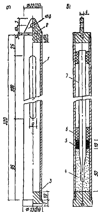
Рис. 6. Конструкция инерционного термометра а - оправа термометра; б - способ придания инерционности термометру; 1 - футляр (винипласт); 2 - заглушка верхняя (алюминий); 3 - заглушка нижняя (алюминий); 4 - изолирующий материал (пенопласт); 5 - гидроизоляция (тиоколовая мастика); 6 - изоляционная лента; 7 - психометрический термометр
