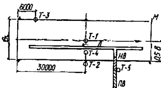
Рис. 1. Расположение температурных скважин и нивелирных марок
