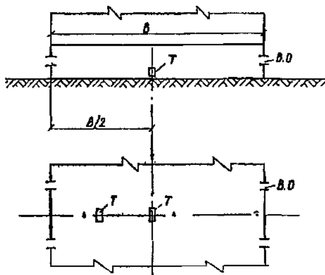
Рис. 8. Схема размещения термографа или инерционного термометра в подполье здания
