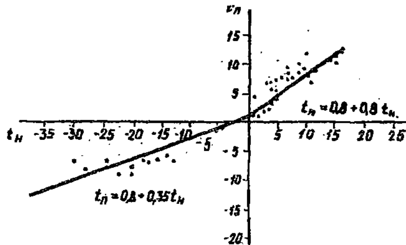
Рис. 10. График зависимости температуры в вентилируемом подполье от температуры наружного воздуха ( A_1 = A_2 )
