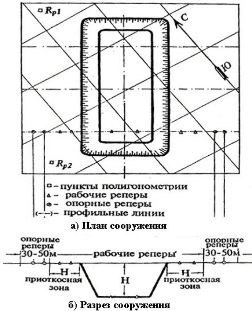
Р и с у н о к У.2 - Схема к составлению проекта размещения реперов при открытом способе строительства подземного сооружения
