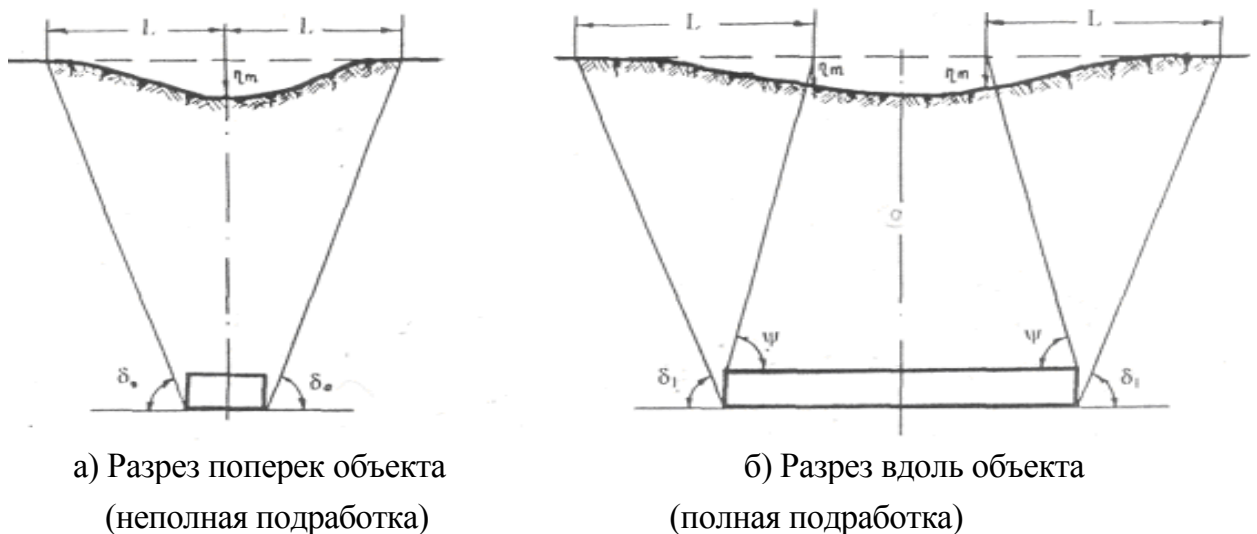
Р и с у н о к С.1 - Основные параметры мульды сдвига
