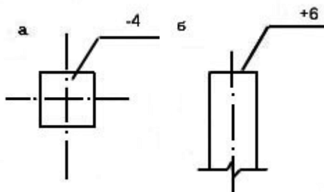
а - сваи или колонны на плане; б - колонны на разрезе
